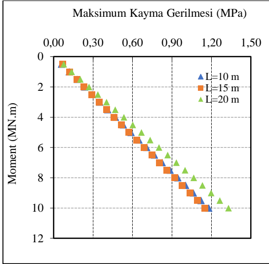
Şekil 8. Farklı boylara sahip kazıkların kayma gerilmesi-moment grafiği
