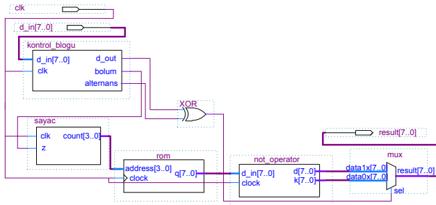
Şekil 5: Önerilen BPSK modülatörün FPGA ortamında tasarımı.
