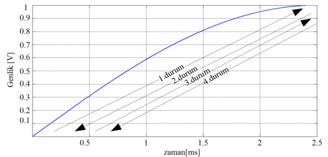
Şekil 7: rom bloğuna kaydedilen sinyal.
