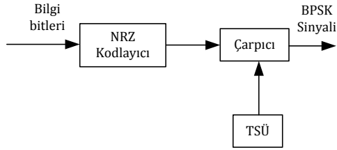
Şekil 1: BPSK modülatör mimarisini.
