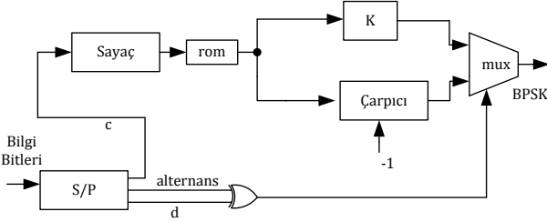
Şekil 4: Önerilen BPSK modülatör şeması.
