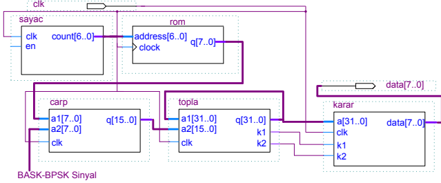
Şekil 8: BPSK demodülatör.
